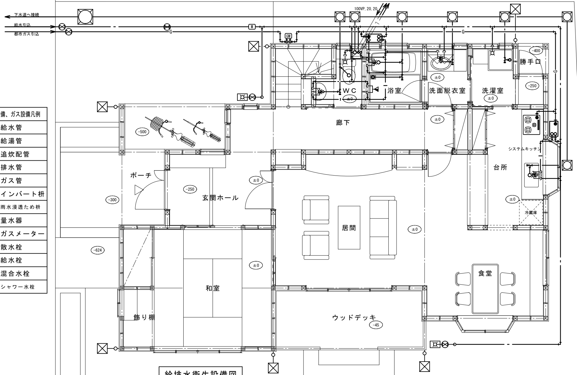
給排水衛生設備図
